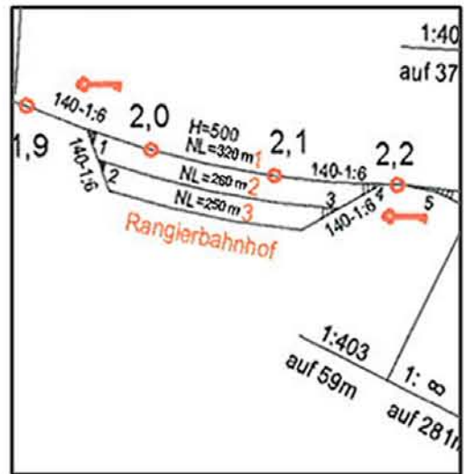
Details Rangierbahnhof
